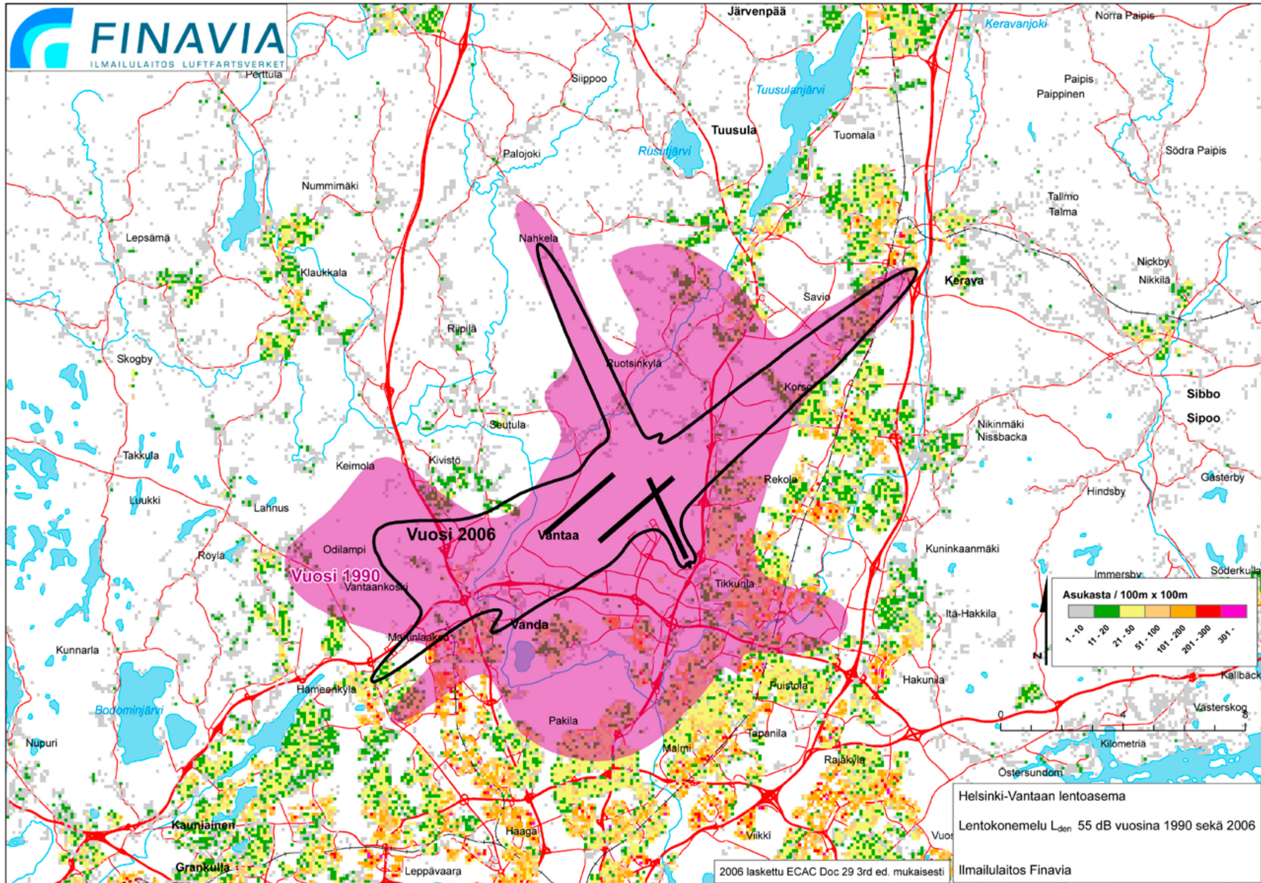
Kuva 5.28 Vuosien 1990 ja 2006 L_{den} 55 dB lentokonemelualueen laajuus. Vuoden 2006 tilanne on laskettu ECAC Doc 29 3rd Edition -menetelmän mukaisesti.
